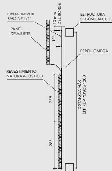
CORTE A-A
